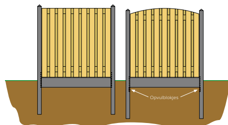
Montage voorbeeld
