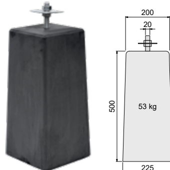
Betonpoer XL
