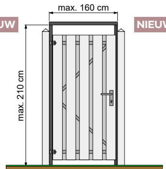
Universeel tuindeurkozijn
